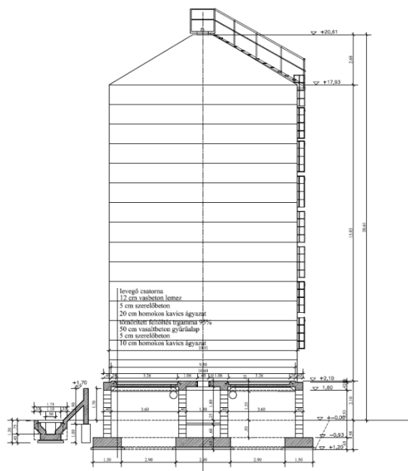
A - A METSZET M 1:100
